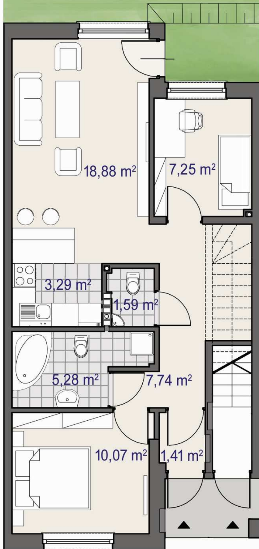
budynek typowy mieszkanie parter 55,51 m 2
