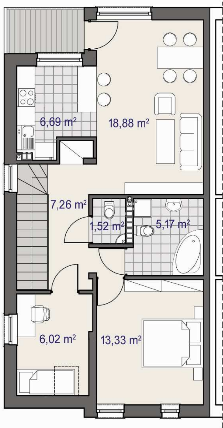
budynek skrajny mieszkanie piętro 64,75 m 2
